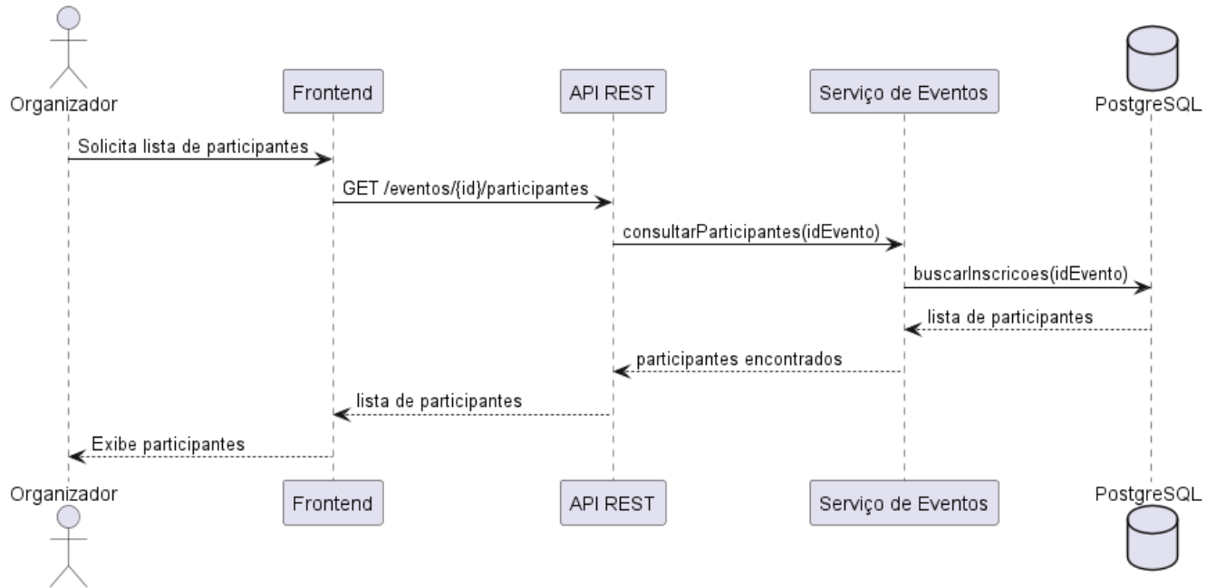
Diagrama de sequência do caso de uso 10:
