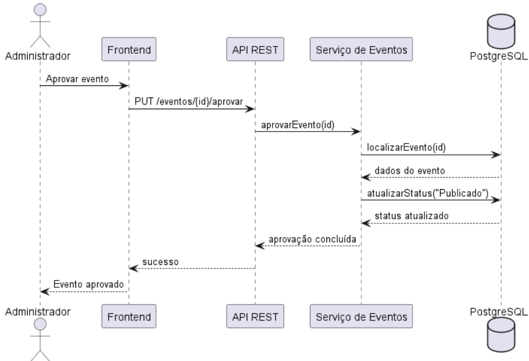
Diagrama de sequência do caso de uso 12:
